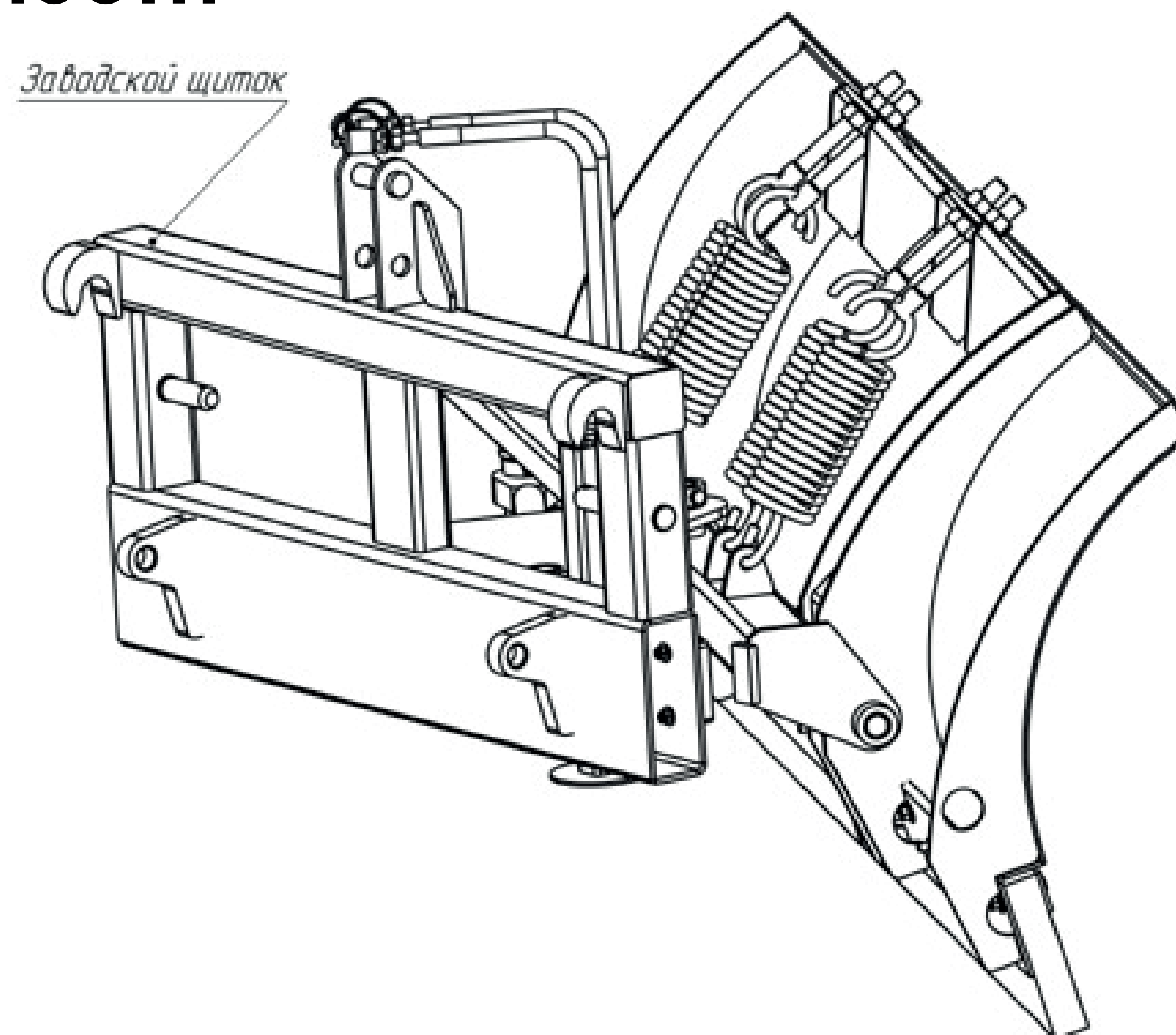
Рис.2. Место крепления заводского щитка на машине
