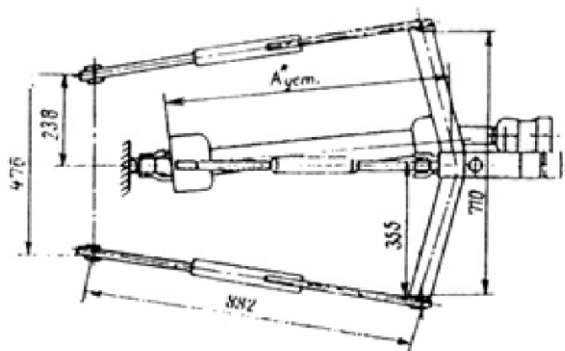
Рис.6 Схема навески косилки на тракторы МТЗ-80 и МТЗ-82.
