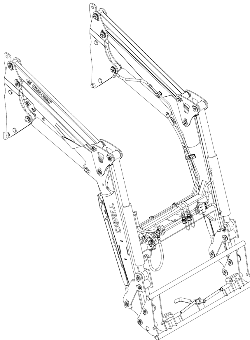
Стрела фронтального погрузчика T220/2 КАТАЛОГ ЗАПЧАСТЕЙ
