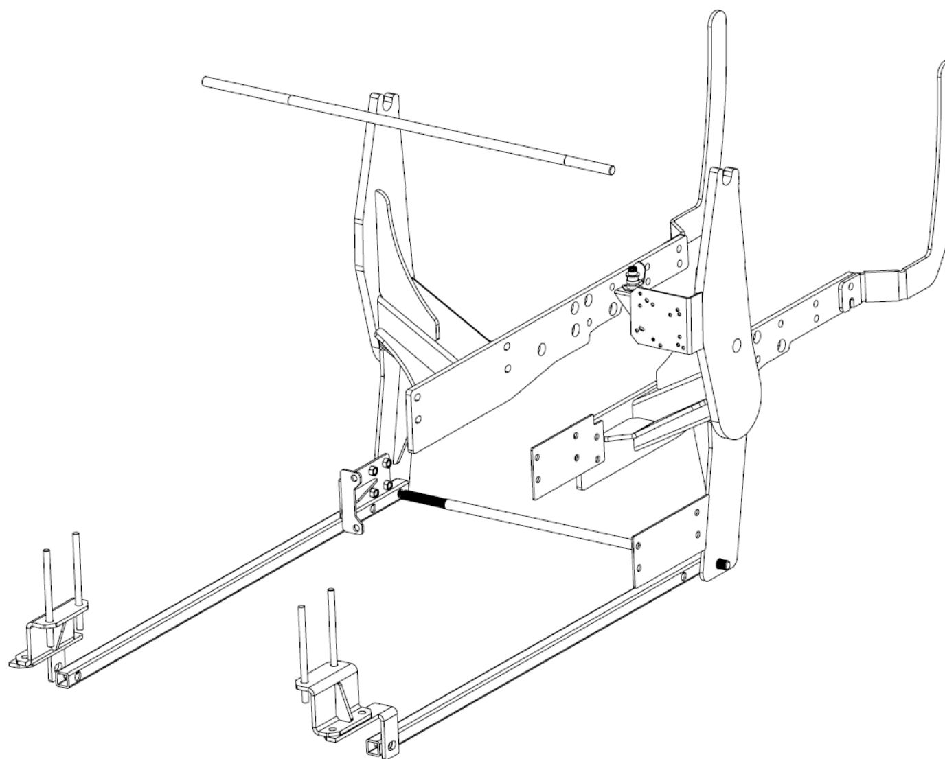
Опорная конструкция T220 к тракторам МТЗ 82.1, МТЗ 82.3 подключение «с кнопкой» КАТАЛОГ ЗАПЧАСТЕЙ
