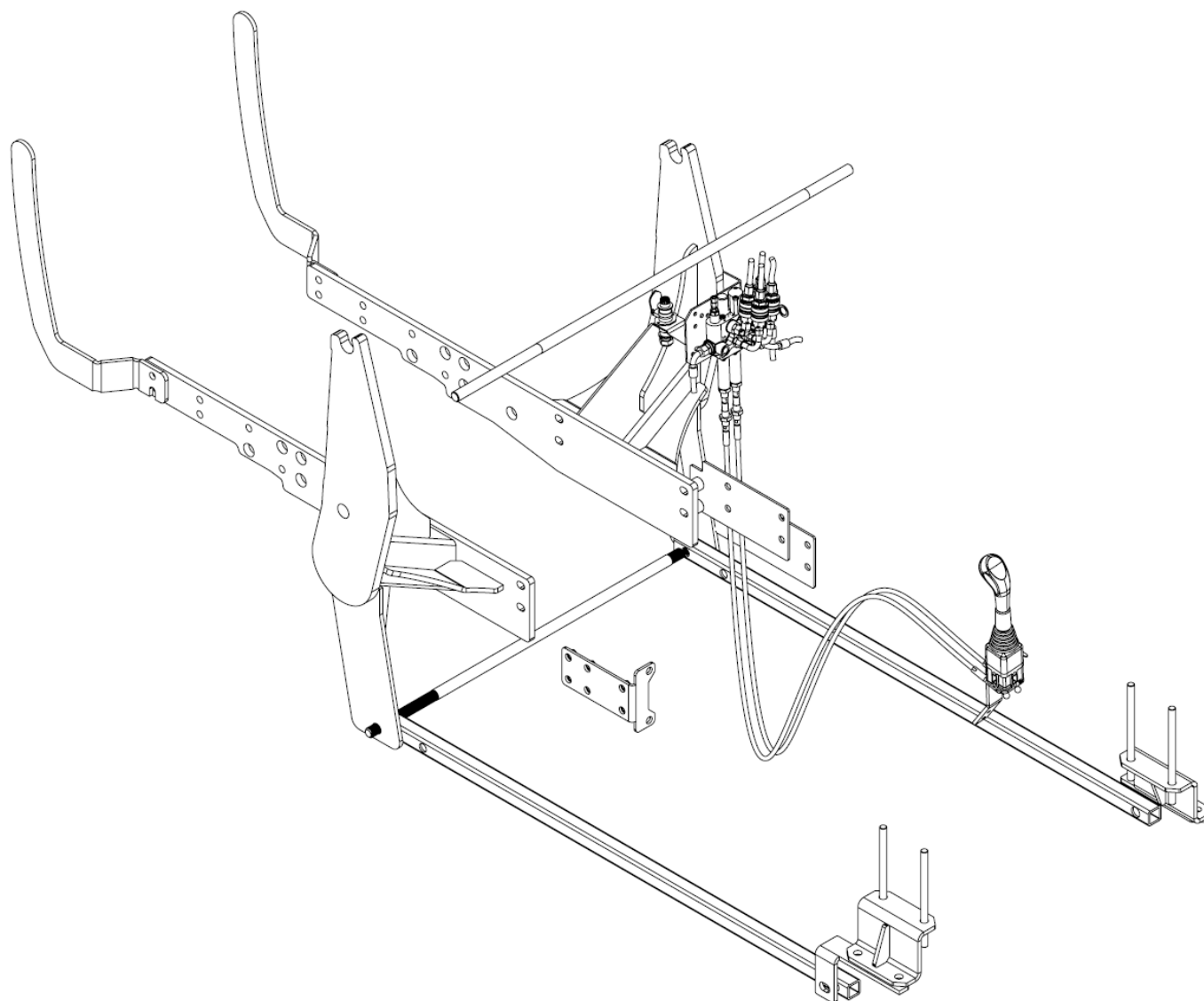
Опорная конструкция T220 к трактору МТЗ 82.1 + МТЗ 82.3 КАТАЛОГ ЗАПЧАСТЕЙ
