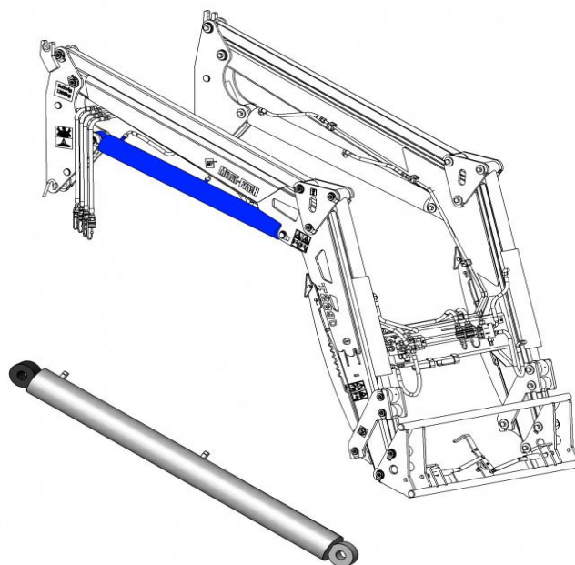
Рис. 9 - Гидроциліндр 70/40/500 S34-р 24SCJ70/40/500 P
