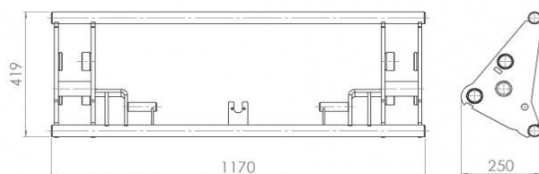
T229-K.080.001.000.2 Рамка поворотная погрузчика T229
