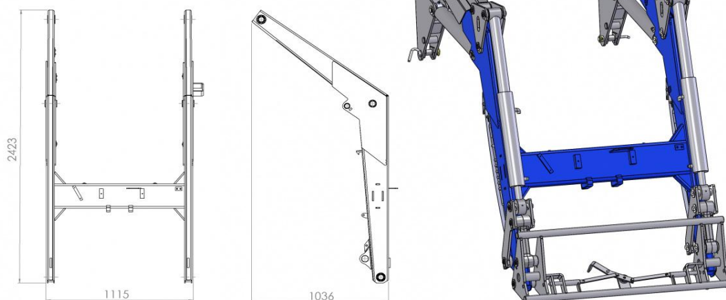
T229-K 180.000.000.2 Стрела сварная погрузчика T229 короткая
