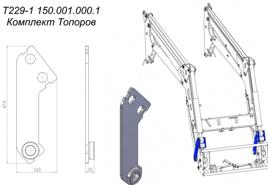
Рис. 6 - Комплект Топоров T229-1 150.001.000.1
