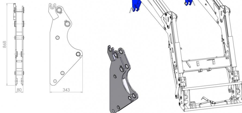
T229-1 012.000.000.3L+P Комплект стоек погрузчика T229
