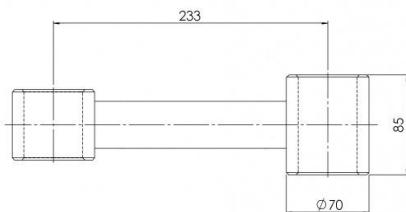
T229-1 010.001.000 Тяга 1
