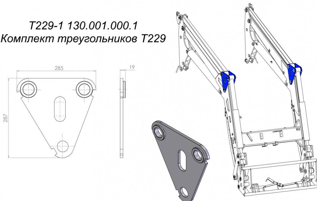
Рис. 4 - Комплект треугольников T229-1 130.001.000.1
