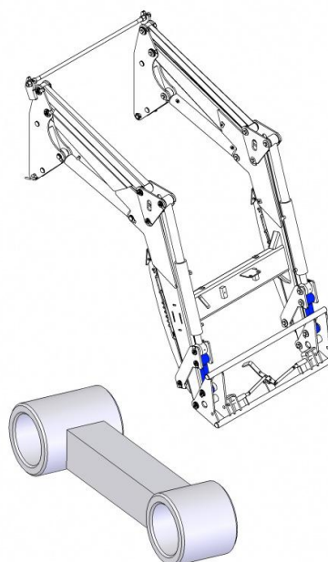
Рис. 7 - Тяга T229-1 010.001.000
