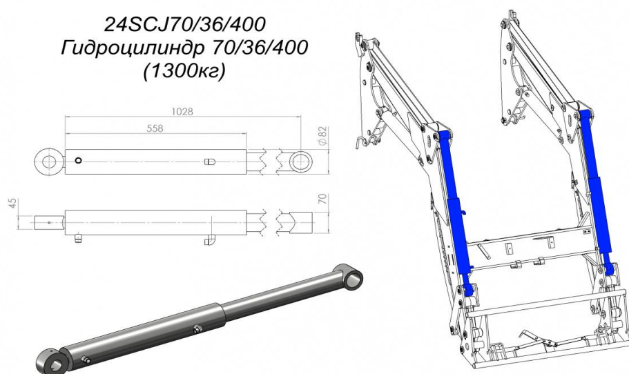
Рис. 5 - Гидроцилиндр 70/36/400 S35 24SCJ70/36/400
