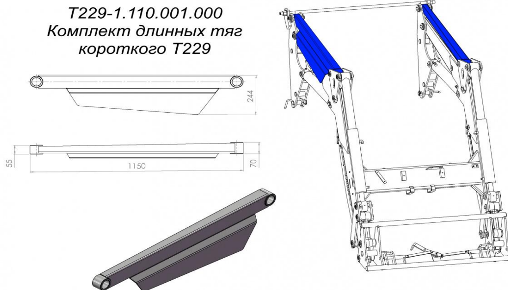
Рис. 3 - Комплект длинных тяг короткого T229 T229-1.110.001.000
