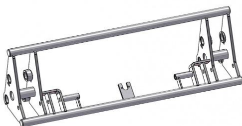
Рис. 8 - Рамка поворотная погрузчика T229 T229-K.080.001.000.2
